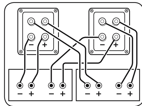
Bi-Amping
